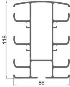
Viga carril S3
