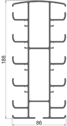
Viga carril S5
