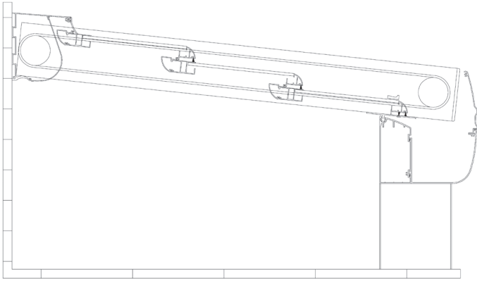
Viga carril S5
